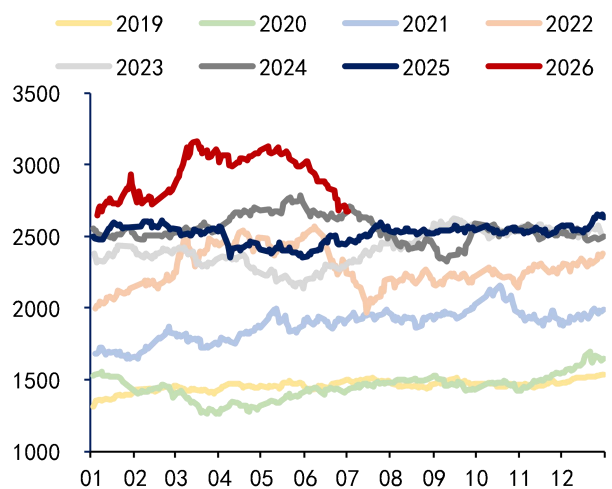
图表 44 南华综合指数
